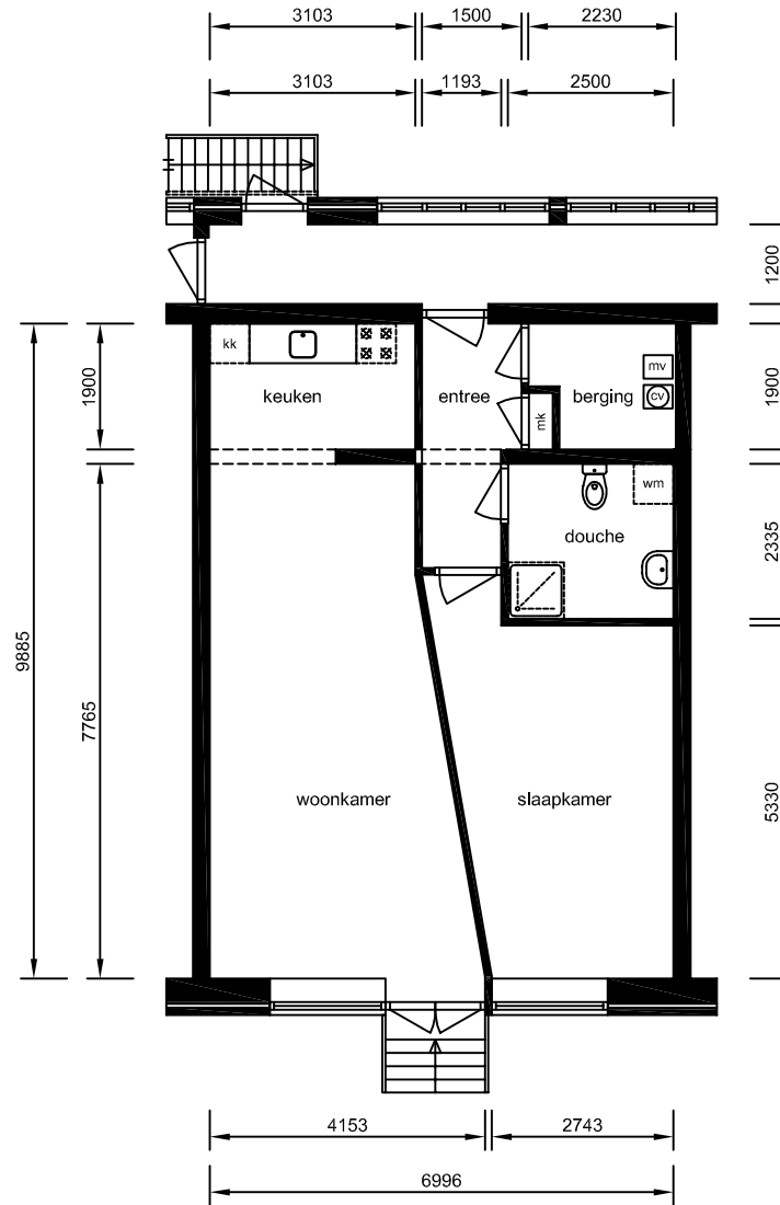
begane grond
